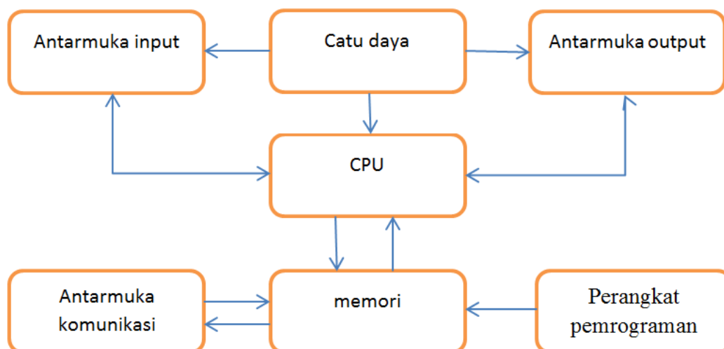
Gambar 1. Komponen PLC
