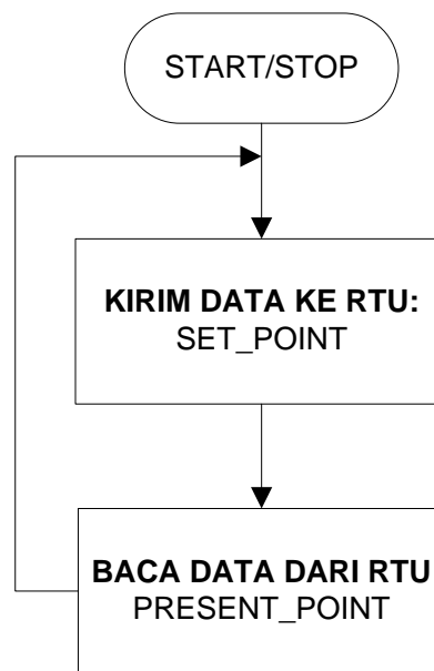
Gambar 6. Diagram alir proses di MTU
