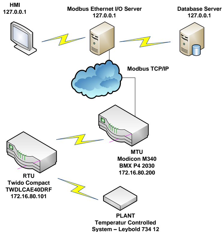
Gambar 2. Arsitektur SCADA
