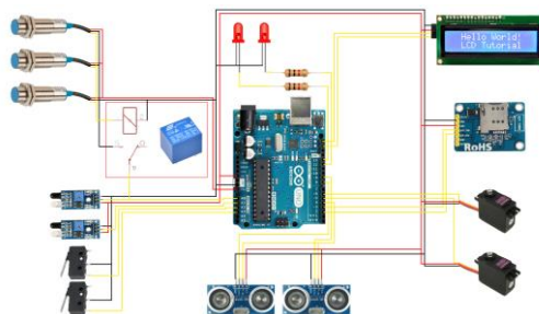
Gambar 3.3 Perancangan Hardware.
