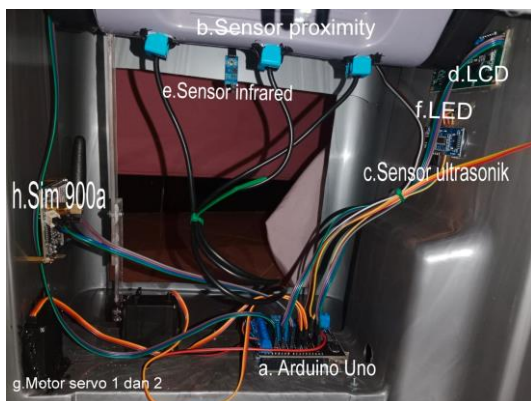
Gambar 4. 1 Rangkaian Keseluruhan.
