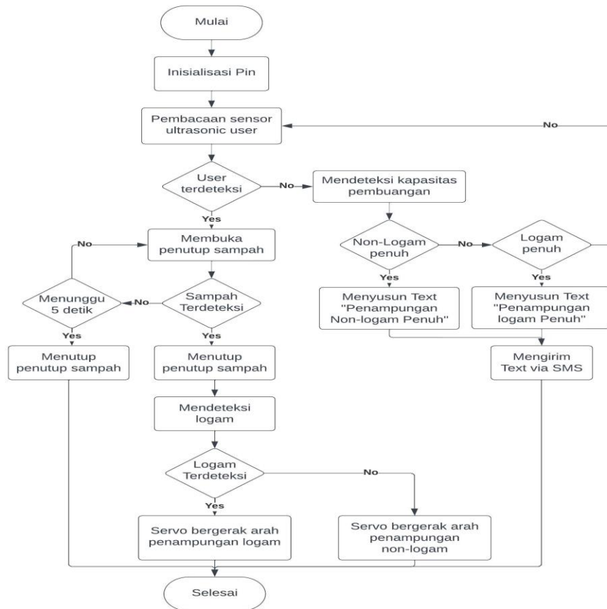
Gambar 3.2 Perancangan Software.
