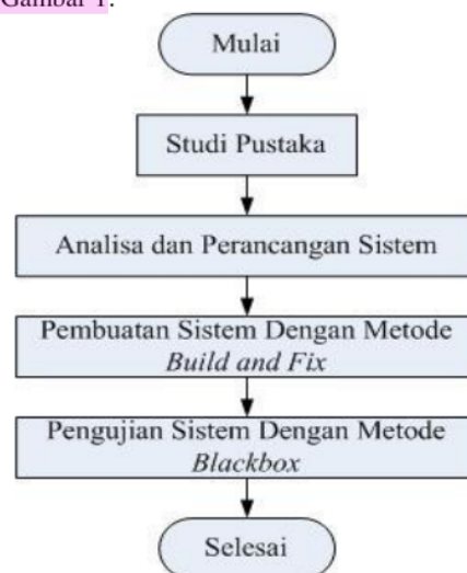
Gambar 1. Tahapan Penelitian
